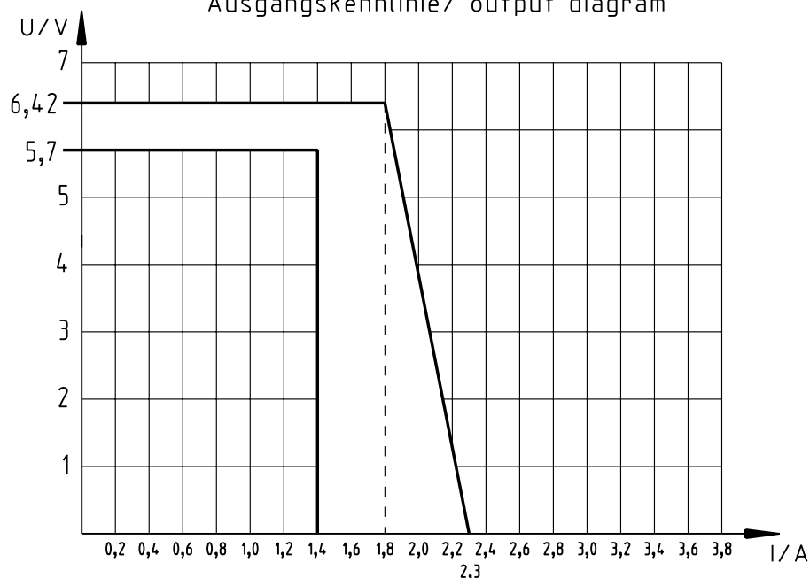
Ausgangskennlinie/ output diagram
