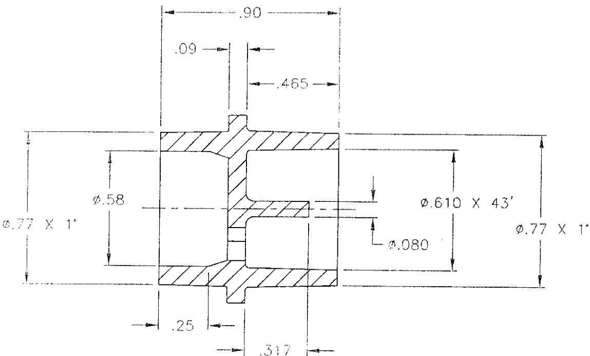
SECTION A--A
