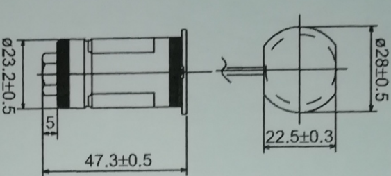
KE-25/KE-50 standard version
