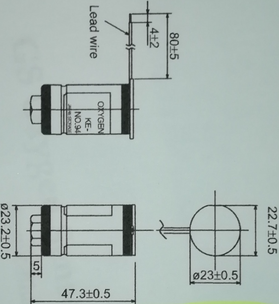
KE-25F1 (w/o flange)
