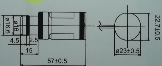
KE-25F4 (O-ring top)
