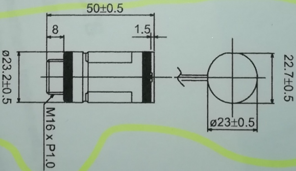
KE-25F3 (threaded top)
