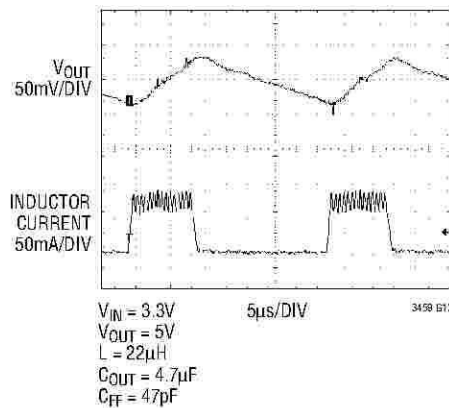
V_{OUT} AC Ripple
