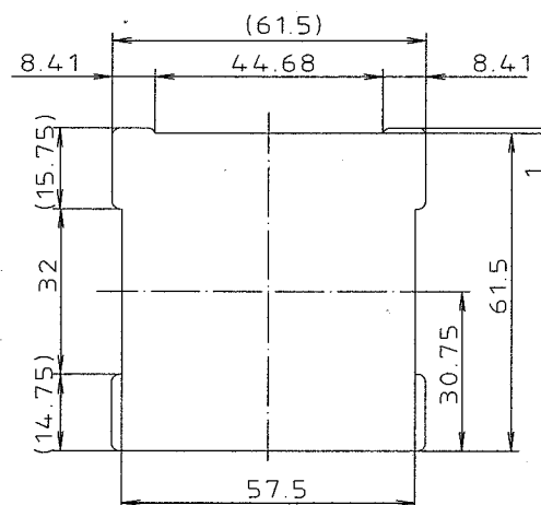
Einbauöffnung BE 60
