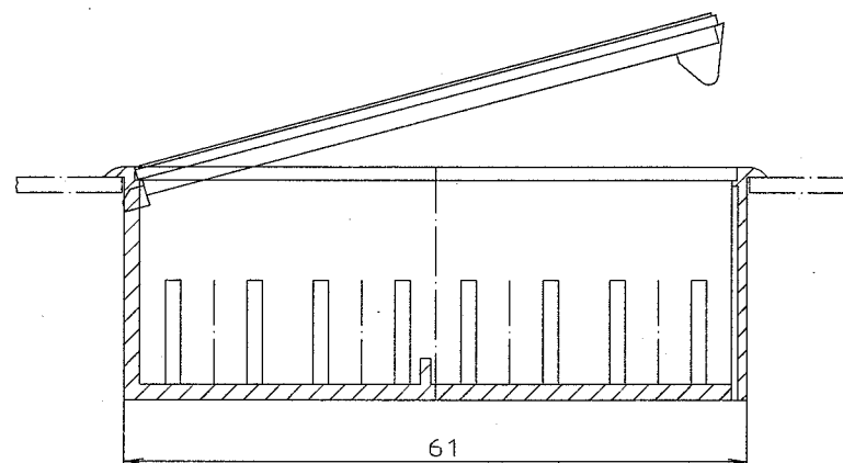
Einbauöffnung BE 60
