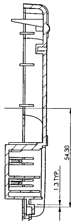
SECTION W-W SCALE 4 : 5
