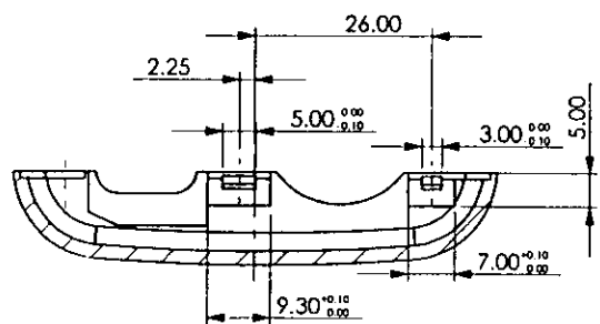
SECTION T-T SCALE 4 : 5
