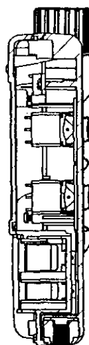
SECTION D-D SCALE 1:2
