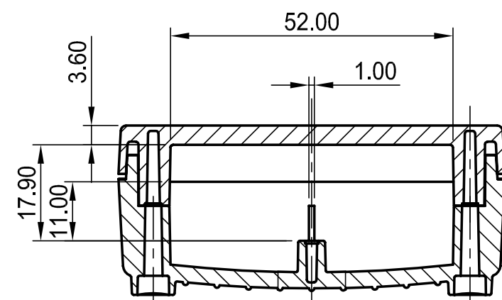
SCHNITT C-C section
