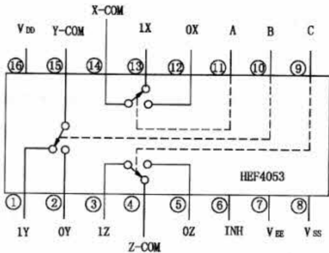
HEF4053 集成块的内电路方框图
