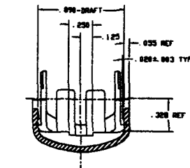
SECTION VIEW B-B (SCALE: 4X)
