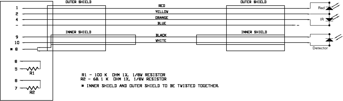
DIN male 8 pin
